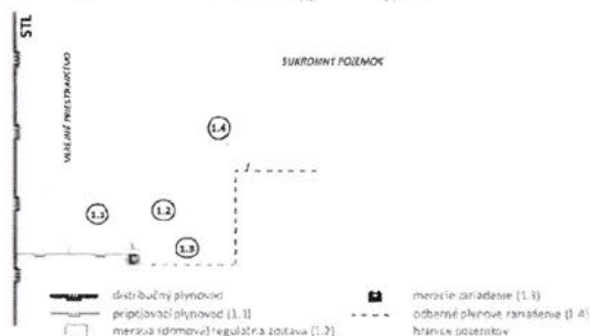
Orientačný náčrt zariadení podľa vyššie uvedenej špecifikácie
