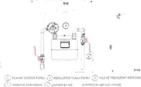
Detail meracej (domovej) regulačnej zostavy
